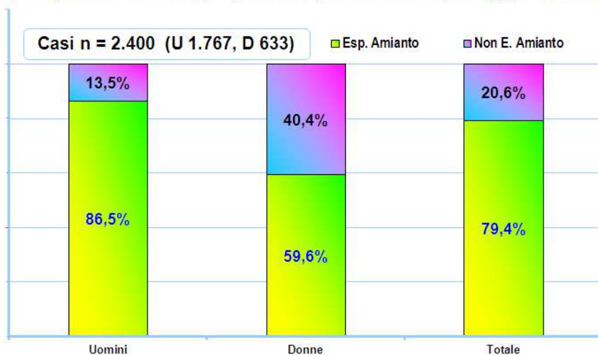
Fig. 3 Esposizione ad amianto per genere in Regione Emilia-Romagna (agg. al 30/06/2019)
