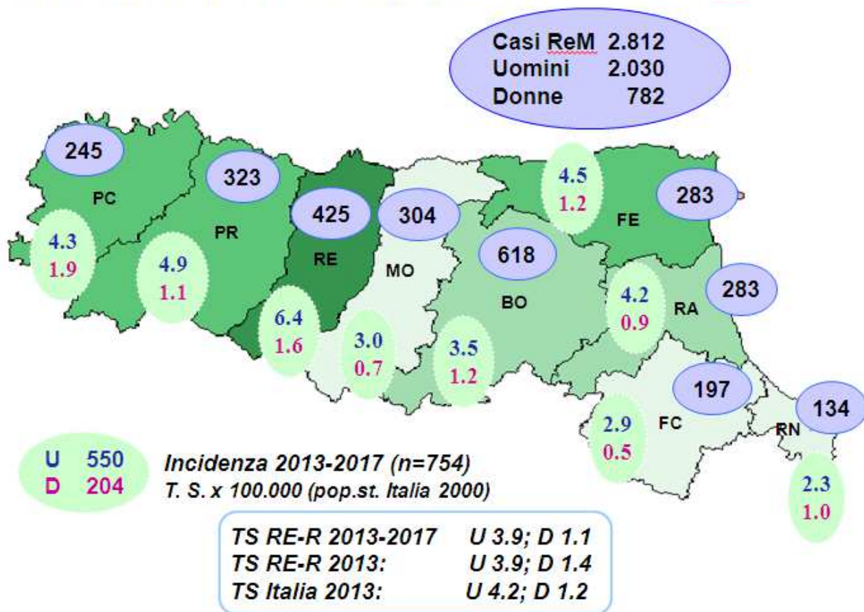
Fig. 1 Distribuzione per residenza: casi incidenti tutte le sedi 1996-2019 (agg. 30/06/2019)
